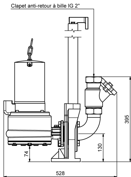
Disposition de montage stationnaire
